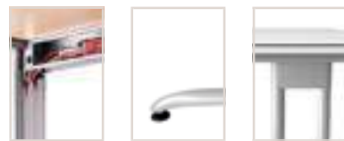
Kabelwanne hor. 8,5 x 9 cm Höhenjustierung +/- 5 mm Stahlrohr Ø3,5/4,7 cm
