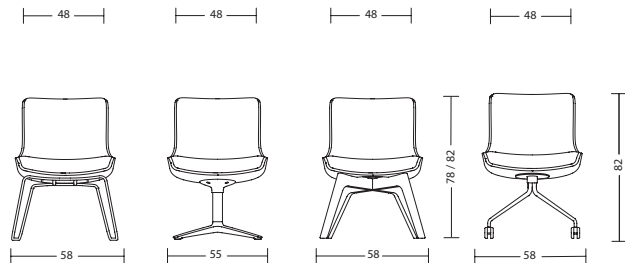
woo56 + 3246 / 3231 / 3206 / 3226 ohne Armlehne: 7 kg
